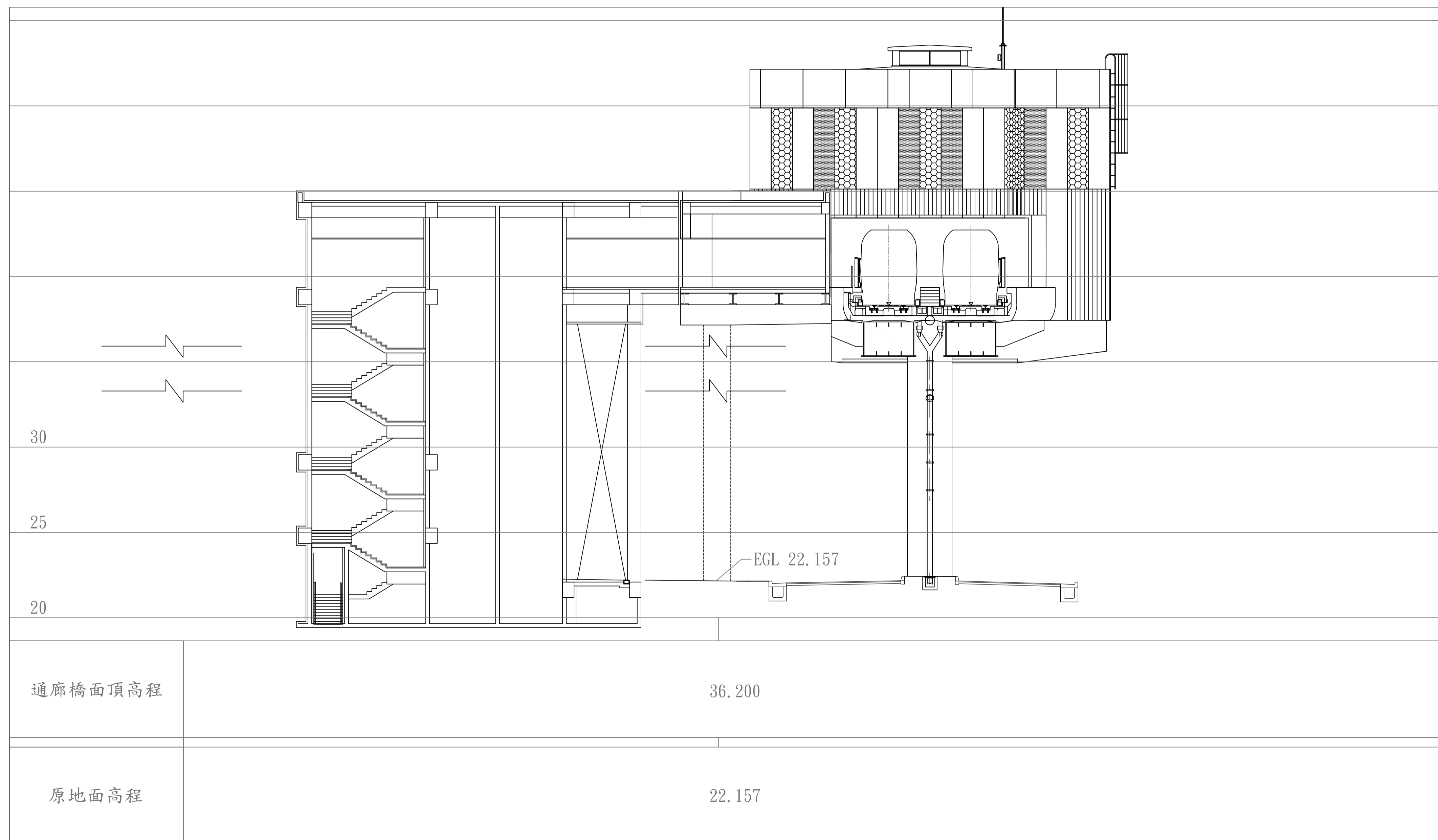
橫剖面圖
